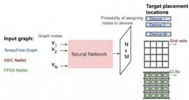
图 | 谷歌自动布局研究(来源:Google Brain)
