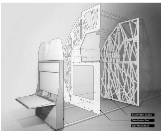
图 | 空客的飞机座椅隔板设计(来源:Autodesk)
