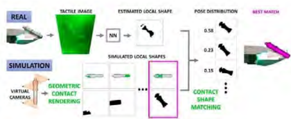
图 | 帮助机器人通过触觉感知来定位物体
