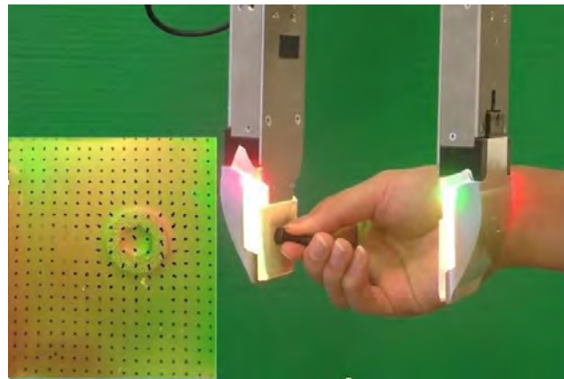
图 | 研究人员使用的触觉传感器
